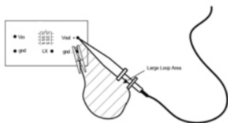
图四(不推荐): 用自带地线夹接被测信号地
