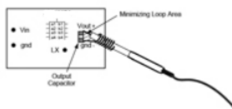
图五(推荐): 探头顶部接地位置接被测信号地
